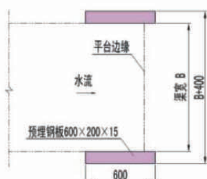
预埋件图
